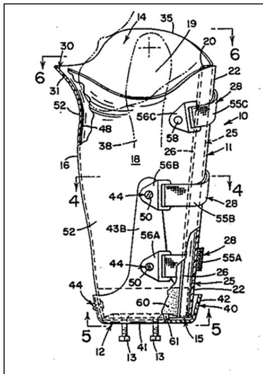
Figura 2:Encaje con contención isquiática anatómica
